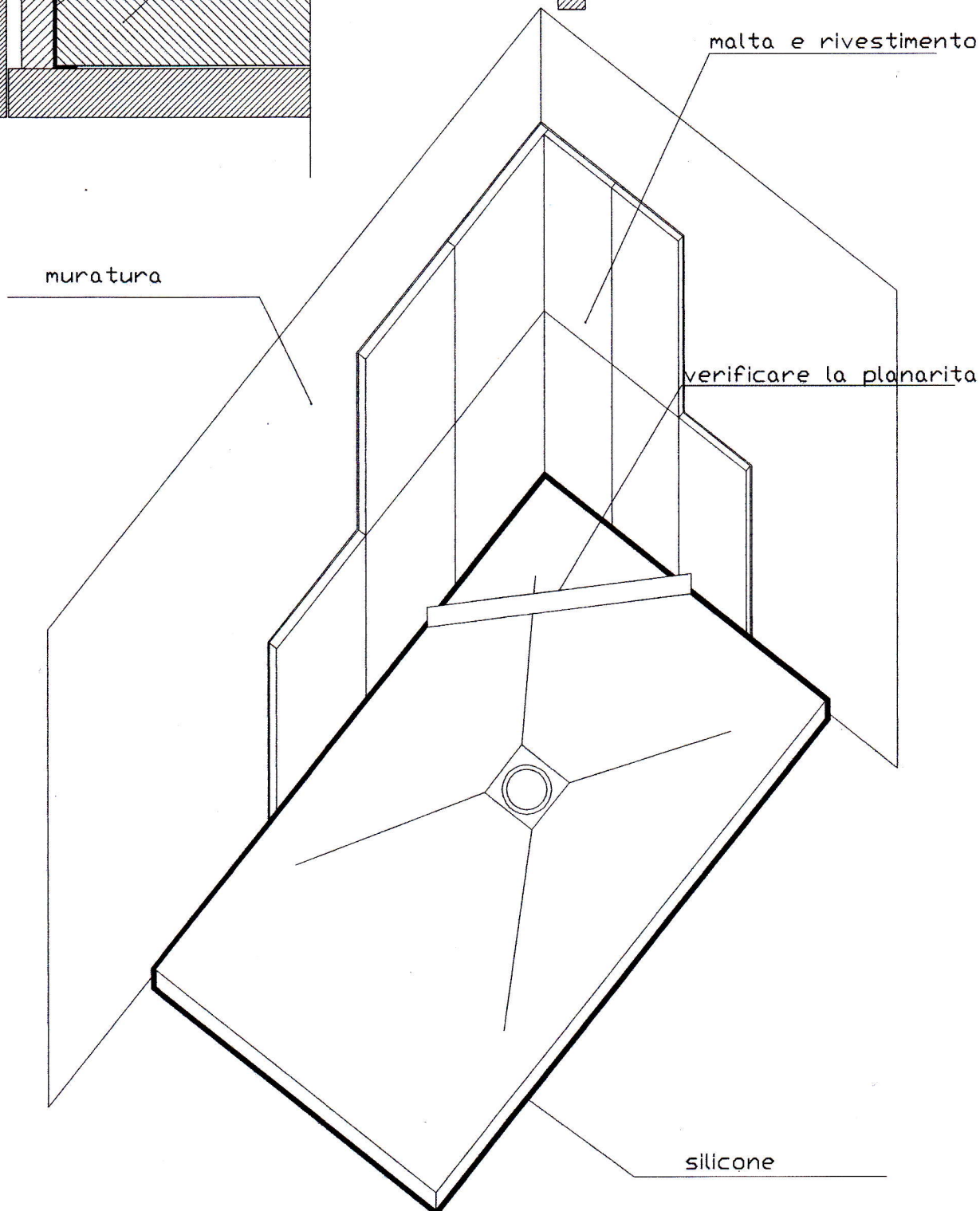
PIATTI DOCCIA WOODY DA 140 FINO A 160 CM SCHEMI DI INSTALLAZIONE
