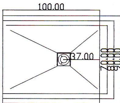
GEOMETRIE DEI PIATTI WOODY
