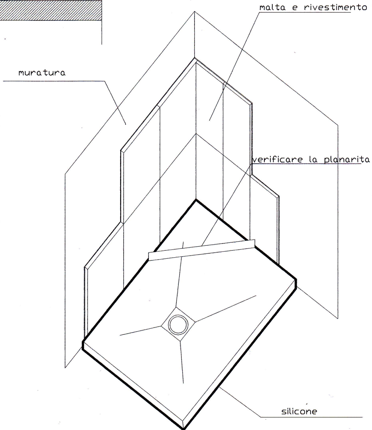
PIATTI DOCCIA WOODY FINO A 120 CM SCHEMI DI INSTALLAZIONE
